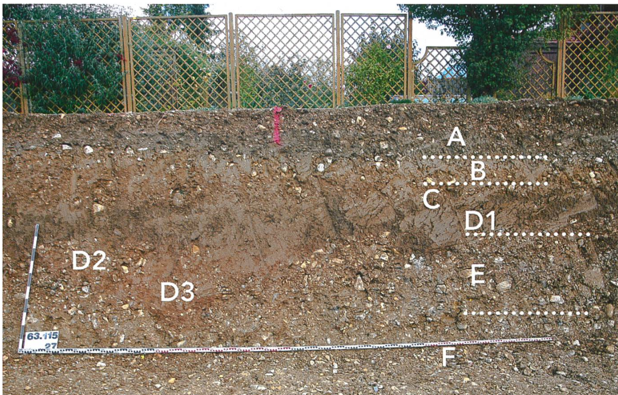
Typische Schichtabfolge in der nördlichen Baugrubenwand (nach Philippe Rentzel).
