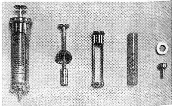
Seringue à injection avec cylindre interchangeable en verre. 2 cc et 10 cc
