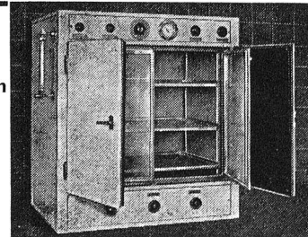
Präzisions-Brutschrank mit Wassermantel und Kühlung
