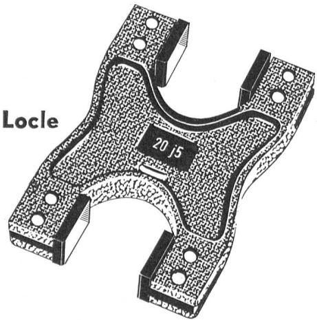
▲ Calibre   m choires en carbure CARY «GIHA» CARY «GIHA» Hartmetall-Grenzrachenlehre
