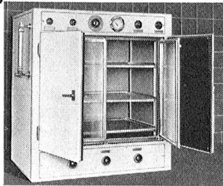
Präzisions-Brutschrank mit Wassermantel und Kühlung
