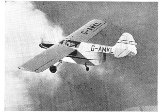
L'appareil Auster B-4. - C'est un avion lent anglais, de création récente. Vitesse: 168 km/h, atterrit à 75 km/h. Il est spécialement conçu pour atterrir sur terrain court (211 m derrière un obstacle de 15 m). Train d'atterrissage très large, souple, de quatre roues, peut être équipé avec skis. Moteur 180 CV, plafond 4000 à 4500 m.
