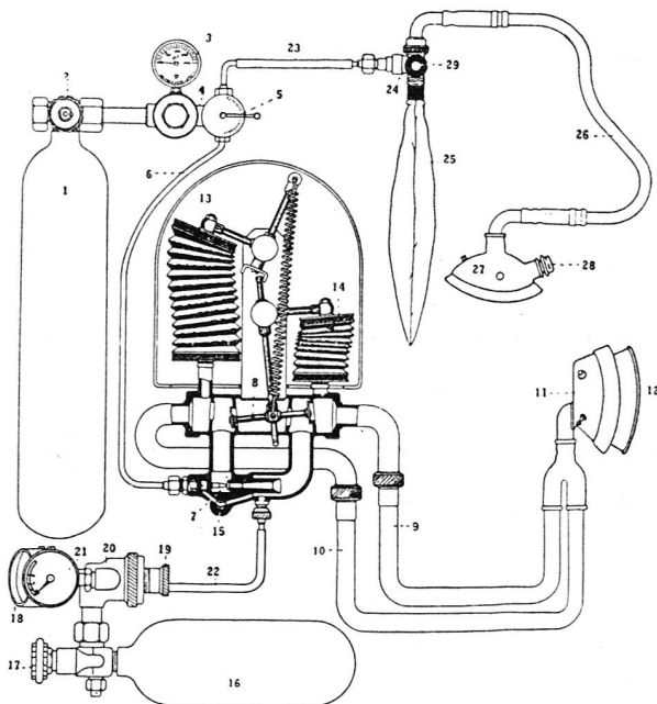
Un pulmotor: 1) bouteille d'oxygène, 6-7) conduite et injecteur d'oxygène, 11-12) prise d'air et tuyaux d'aspiration et d'expiration (8-9), 16) bouteille de gaz carbonique, 26-27) masque de caoutchouc avec valve d'expiration (28). (D'après Rettungsschwimmen , édition S. S. S.)
