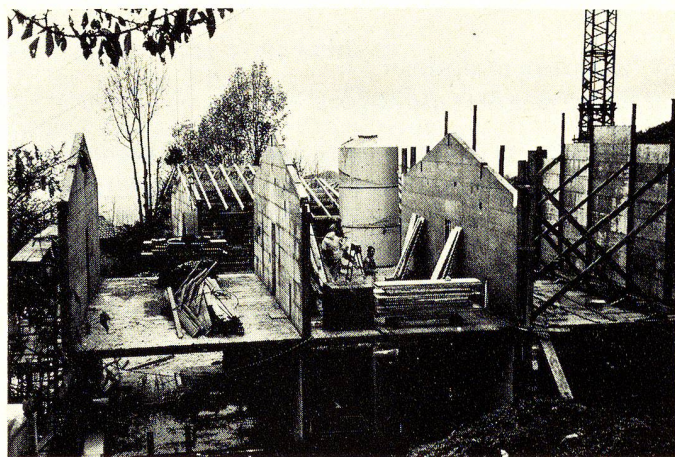
Bien que l'on ait mis l'accent sur la solidité des bâtiments dont seuls les toits, les portes et les fenêtres ont été préfabriqués en Suisse, le prix de revient est resté stable, environ Fr. 120.– le m 3 .
