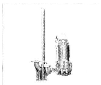
Pompes pour eaux fécales
