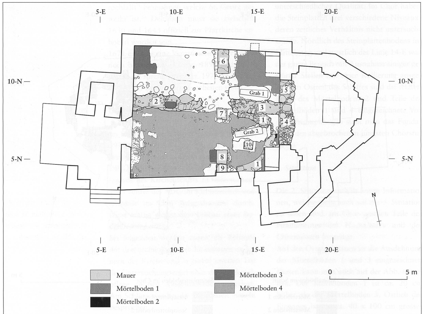
Abb. 58: Schlans, Kirche St. Georg. Grundriss 3. Situation. Mst. 1:150.
