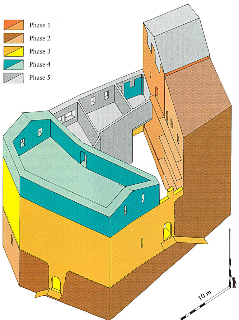
Abb. 214: Brienz/Brinzauls, Burgruine Belfort. Die Burganlage Belfort mit den Um- und Ausbauphasen 4 und 5. Schematische Isometrie von Südosten. Mst. 1:400.
