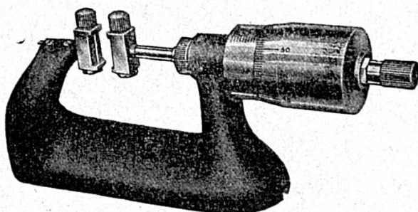
MICROMÈTRE pour mesurer les diamètres sur flancs des vis au moyen de 3 fils.
