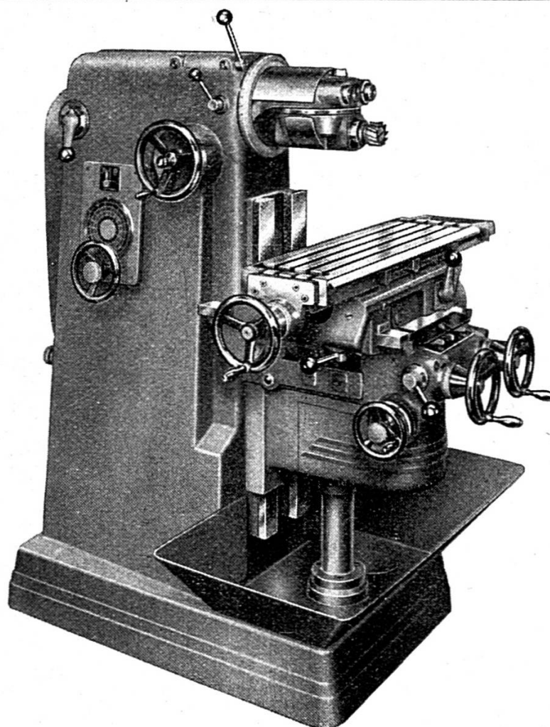
Fraiseuses universelles de grande précision SV 51 / SV 53 Surface de la table 800×215 1100×255 mm
