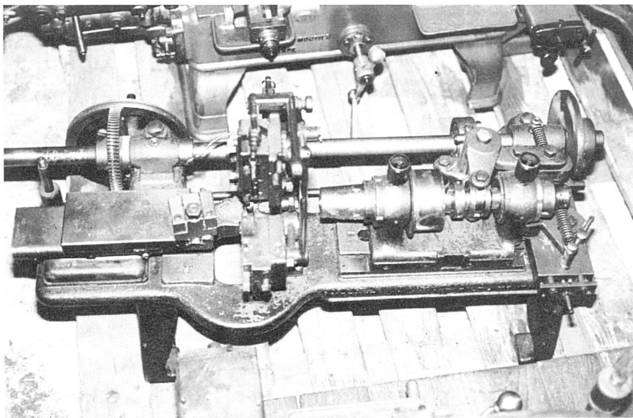
Tour à plateau Mettetal, Junker & C e , 1903. Les principaux organes (arbre à cames, poupée mobile) sont disposés de manière analogue au tour Schweizer conçu avant 1880 (photo d'une machine faisant partie du futur Musée du tour automatique de Moutier).
