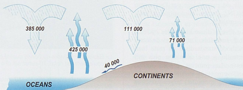
Flux hydriques annuels (en km³) sur l'ensemble de la planète (modifié d'après CNRS).
