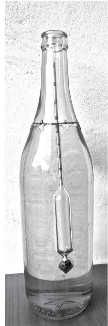
Pèse-alcool.
