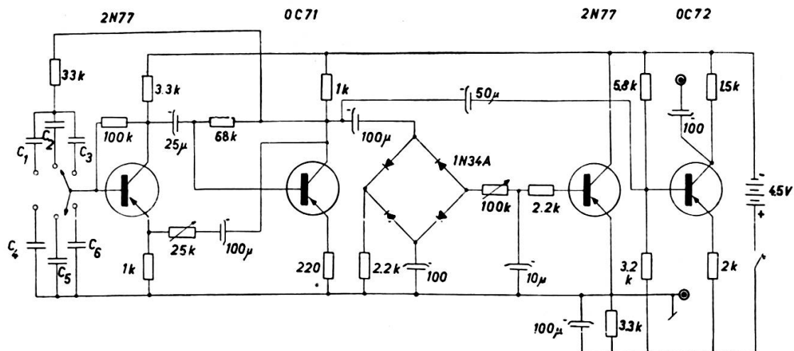
Oscillateur BF
