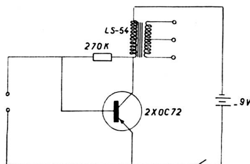
Étage BF de sortie
