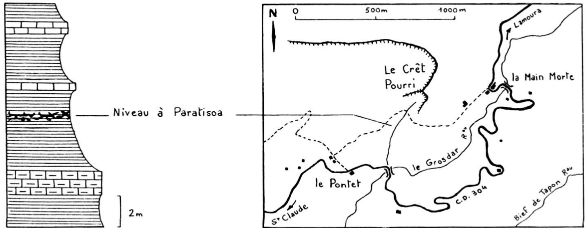
FIG. 1 — Situation du gisement type.
