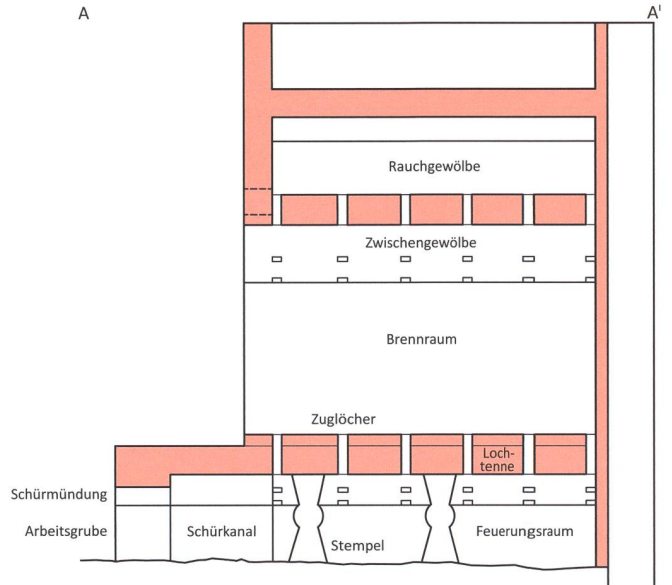
Längsschnitt A-A'
