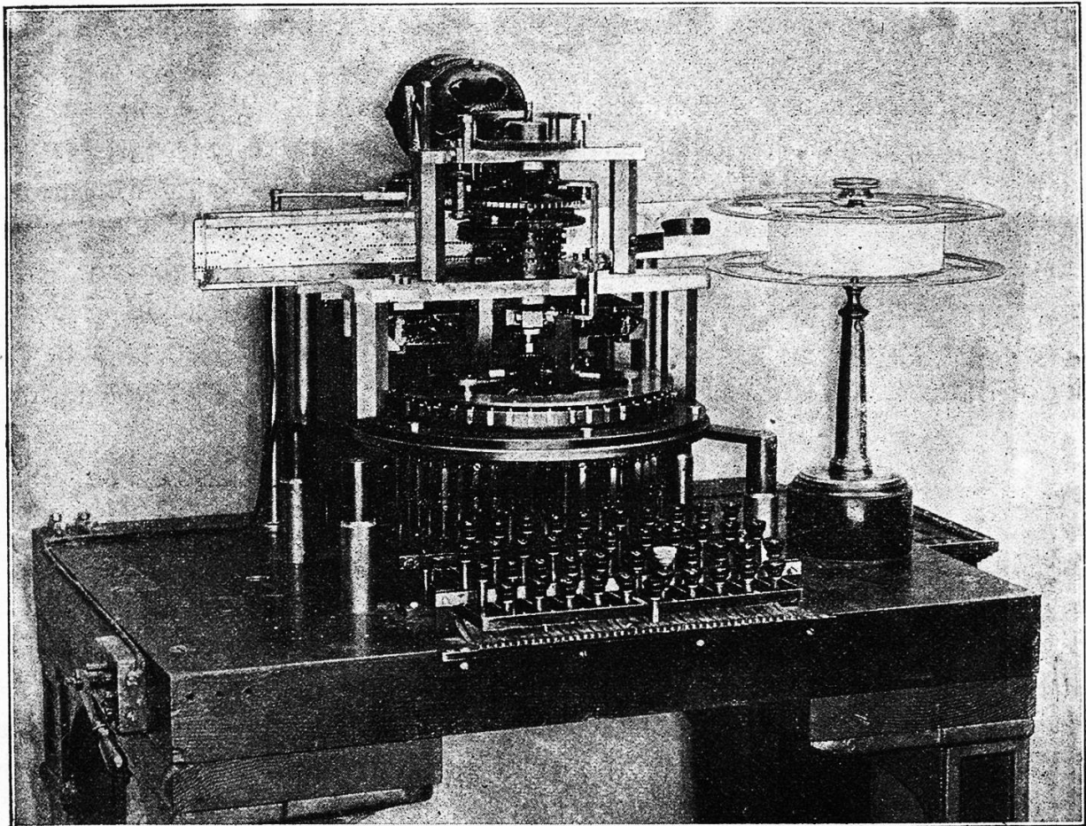
Der Typendruck = Schnelltelegraph. Schreib- und Lochapparat.
