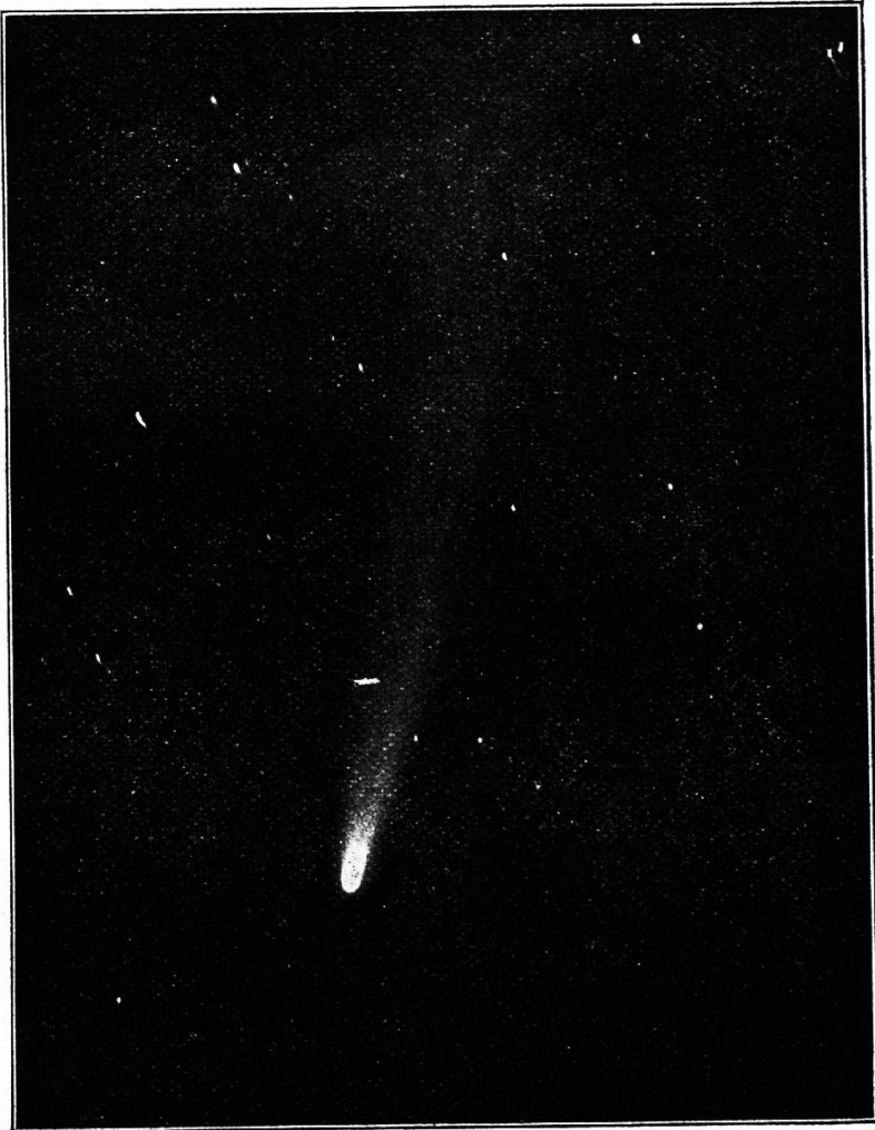
Abbild. 8. Photographie des Kometen Halley, 6. Mai 1910.
