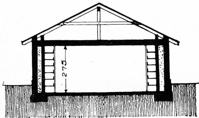
Abb. 4. Obstellagerhaus (Querschnitt).
