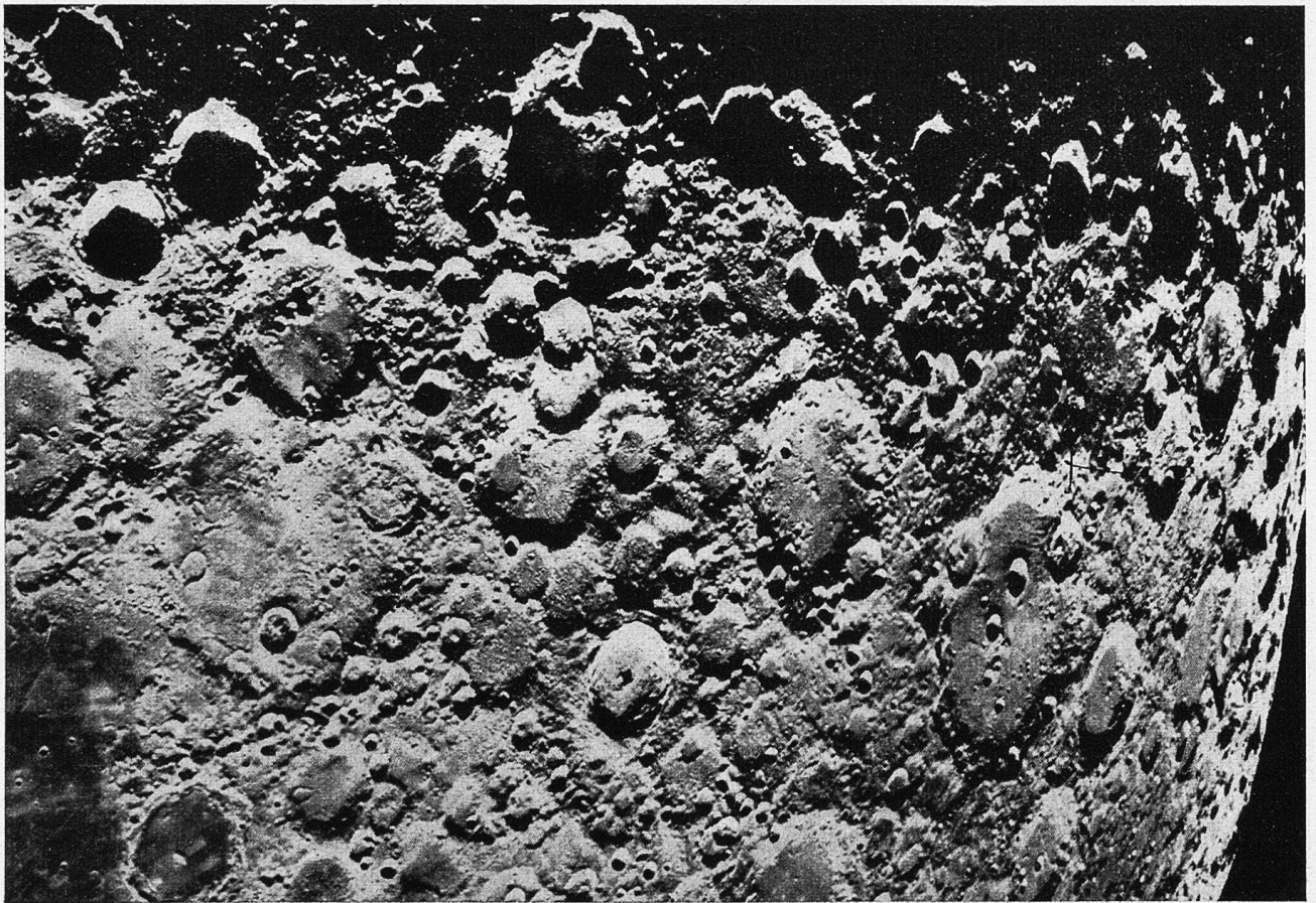
Mondlandschaft. Südlicher Teil der Mondscheibe im letzten Viertel (Mt. Wilson-Sternwarte, Spiegelteleskop von 260 cm Öffnung). Ein ungeheures Gewirr der Gebirgsformen tritt in Erscheinung. Eine wichtige Gesetzmäßigkeit kann dem Beschauer nicht entgehen: die Ringformen kleinerer Abmessung sind stets auf die größeren aufgesetzt. Die letzteren sind also ältere Bildungen.
