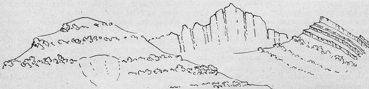
Gipfelformen der Nagelfluhberge bei verschiedener Schichtlage (nach Albert Heim)
