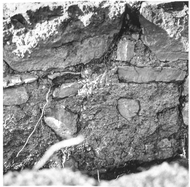
Abb.98: Därstetten, Ruine Weissenburg. Originaler Verputz am Donjon.
