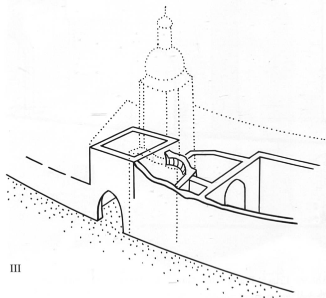
Abb.100: Laufen, Christkatholische Pfarrkirche St. Katharina. Nordfas- sade mit Stadttor und Eintragung baugeschichtlicher Befunde. M. 1:200.
