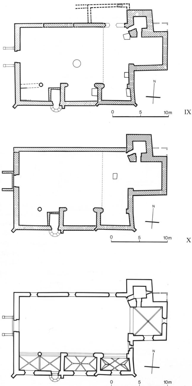
Fig.111: La Neuveville, Blanc Eglise. Plans des différentes dispositions. Echelle 1:400. Vestiges profanes et les églises (I-X).
