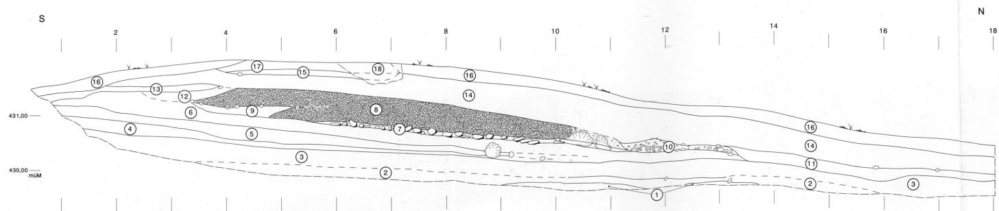
Abb. 18: Leuzigen-Matte 1990. Profil 3. Schichtenbescrieb siehe Text. M. 1:50.
