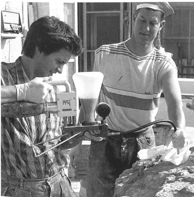
Abb. 15: Laufen - Dolmengrab. Restaurierung 1990/91. Westplatte (12). In die mächtige Kalksteinplatte wird zur Festigung mittels Pumpe Kunstharz injiziert.
