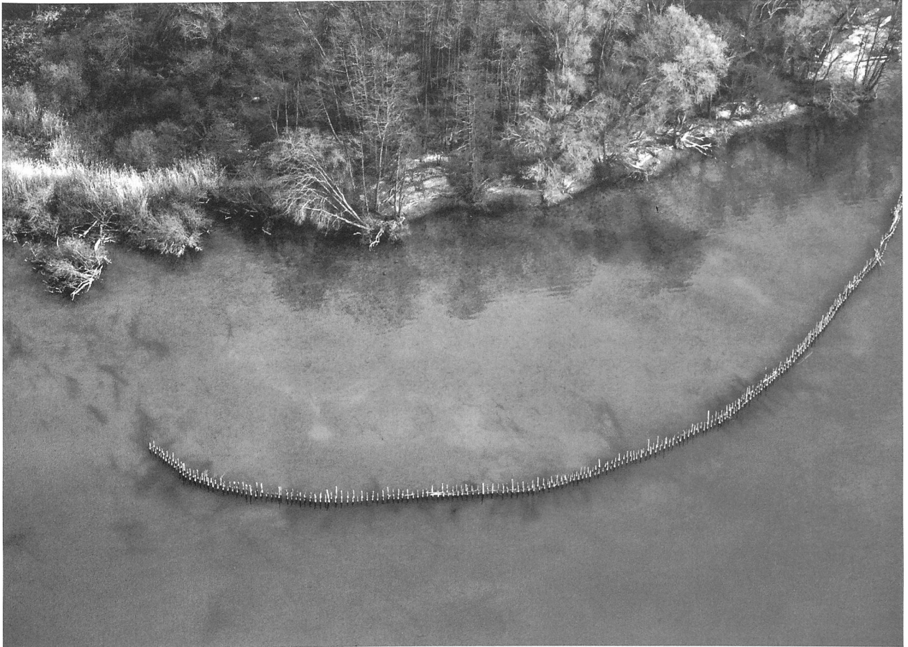
Abb. 59: Sutz-Lattrigen - Rütte 1998. Bau des Wellenbrechers. Die Doppelpfahlreihe für die Lahnung wurde in den Wintermonaten erstellt. Blick nach Osten.
