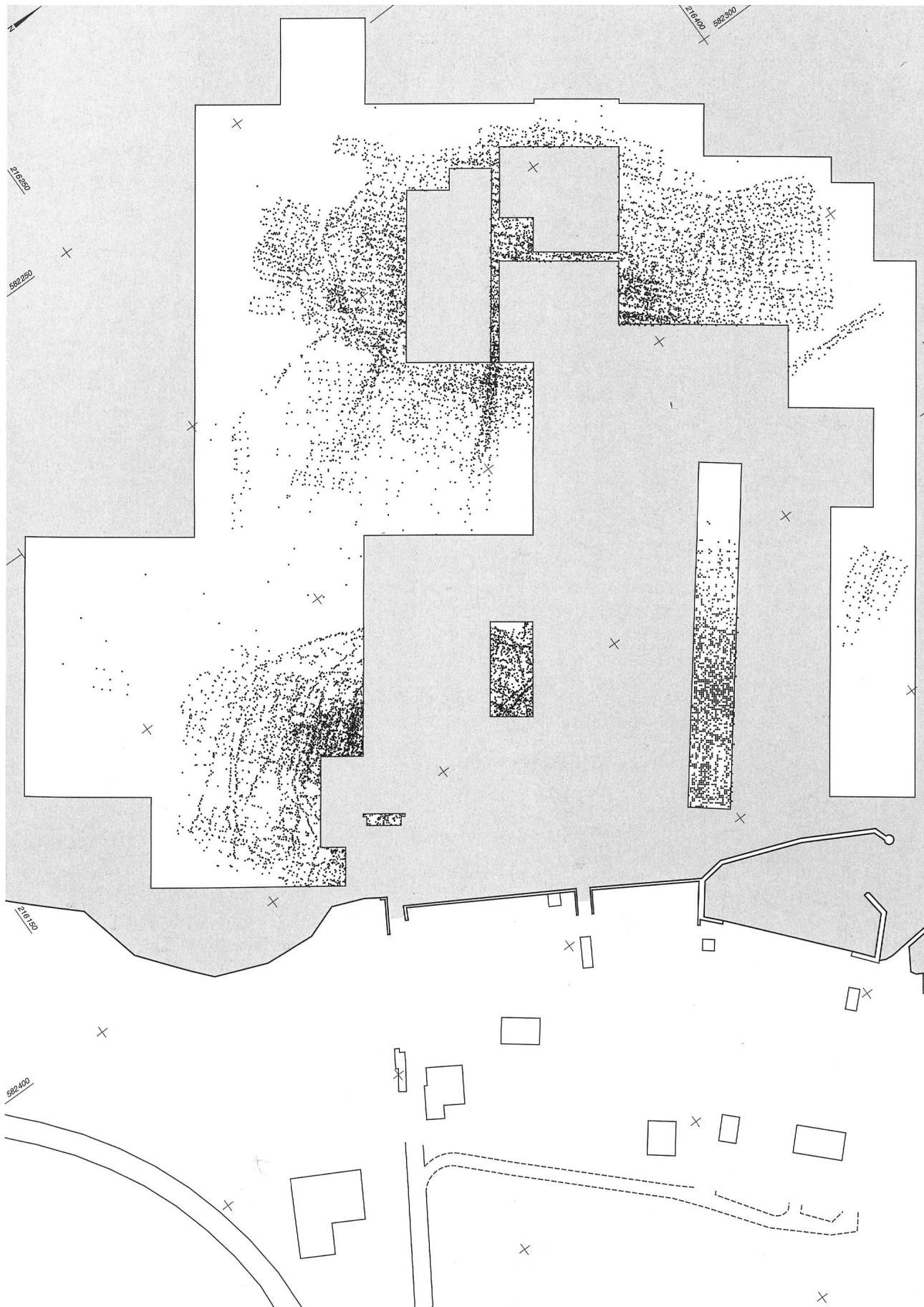
Abb. 38: Sutz-Lattrigen - Hauptstation 1988–2003. Pfahlplan. M. 1:1250
