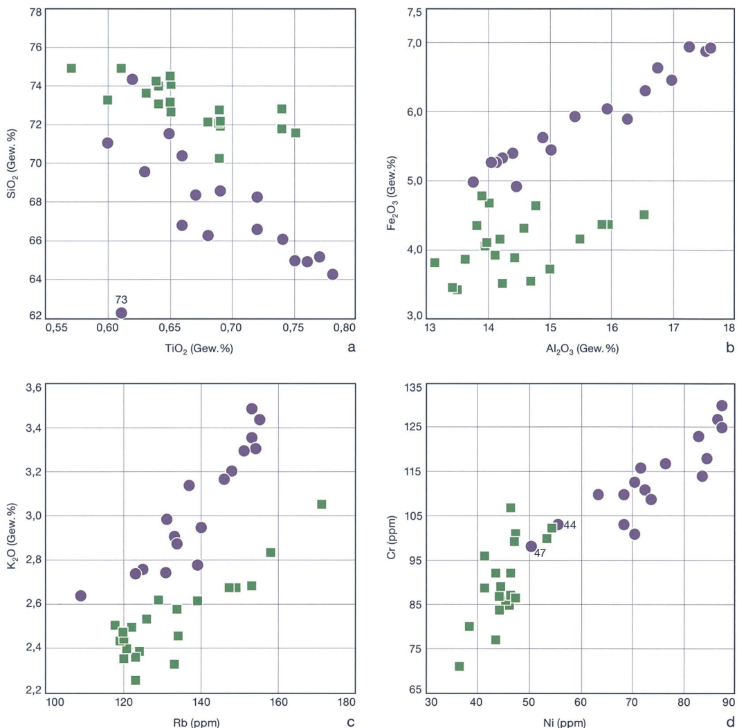
Abb. 8: Vergleich der 17 kantonalbernerischen Ofenkacheln mit denjenigen der Zuger kalziumarmen Referenzgruppe «Hafnerei Oberaltstadt 3/4» (letztes Viertel des 16. Jh., 21 Proben; Zug 1–6, 8–22; Thierrin-Michael 2016).
