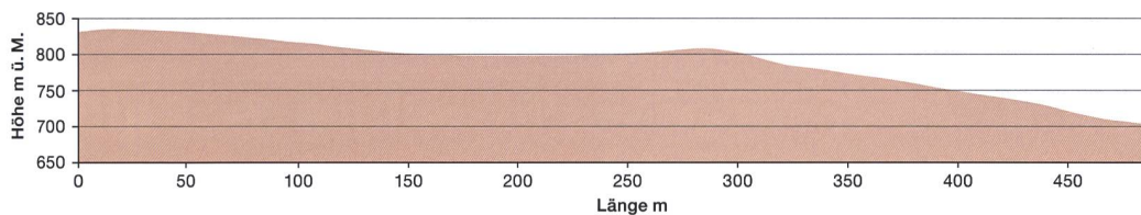
4 Lützelflüh, Grosshus. Geländeprofil Nordost durch den Abhang. M. 1:5000.
