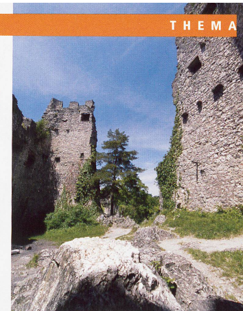
Burgruine Pfeffingen
