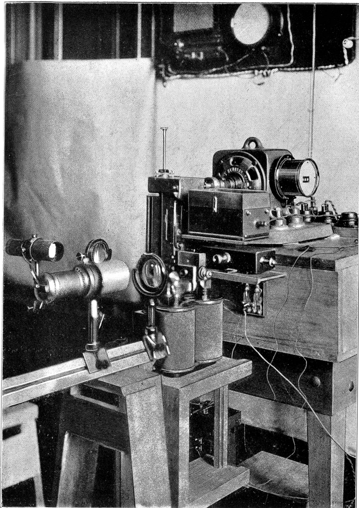
Abb. 2. APPARATUR NACH PROFESSOR KORN (EMPFÄNGERSEITE)
