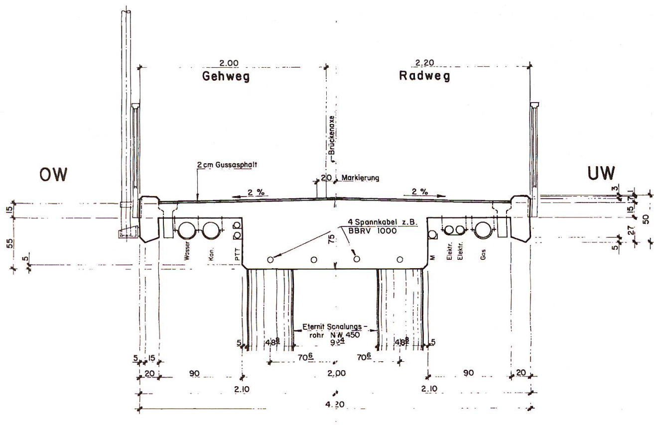
Querschnitt 1 : 20
