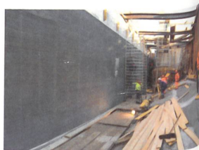
Die horizontal gerichteten Lamellen erzeugen eine für die Stromproduktion und die Lenkung von Fischen optimale Strömung. (Foto: Thomas Stucki)
