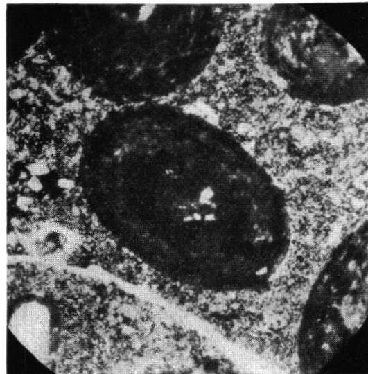
Oolith mit Quarzkern
