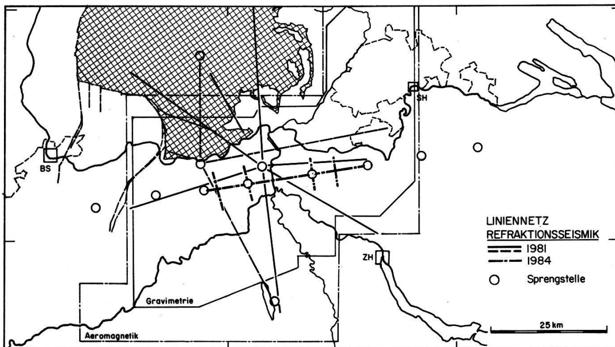
Figur 2: Geophysikalische Untersuchungen der Nagra in der Nordschweiz, 1981–1984, Gravimetrie, Aeromagnetik und Refraktionsseismik
