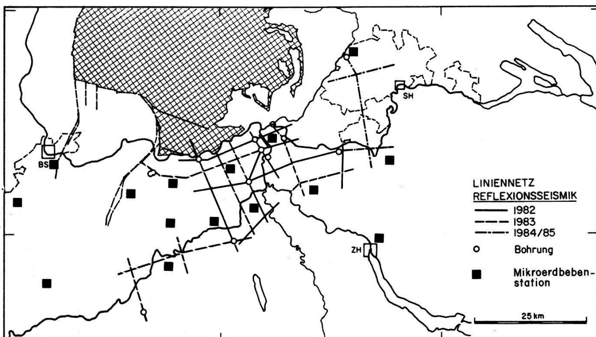
Figur 3: Geophysikalische Untersuchungen der Nagra in der Nordschweiz, 1982–1984/85, Reflexionsseismik und Mikroerdbebenetz
