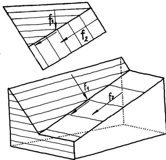
Fig. 45 Modelle von konkaven Gehängen
