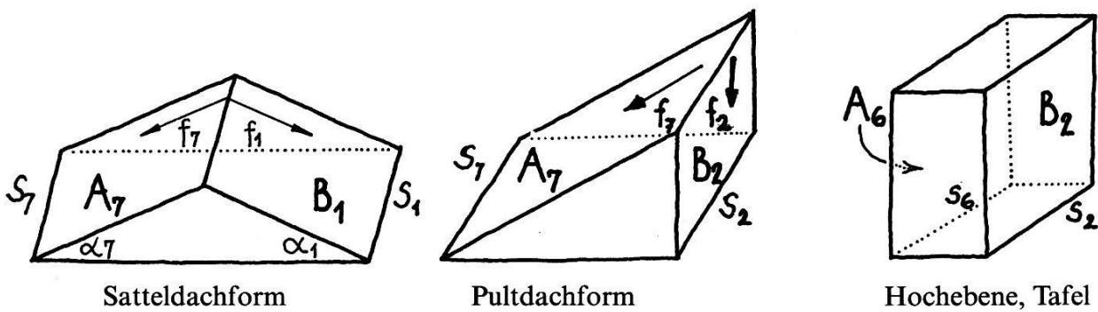
Fig. 32 Typen von Wasserscheiden
