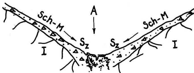
Fig. 80 Talboden aus Gehängeschutt und Geschiebe des Talgewässers A Gewässer-Aufschüttung Sch-M Schuttmantel S z Talboden-Aufschüttung durch das Gehänge I Innengestein
