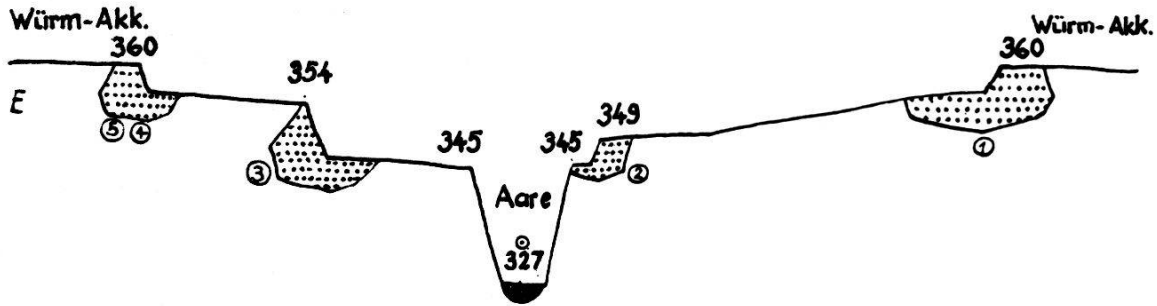
Fig. 87 «Querprofil Würenlingen–Villigen (halbschematisch). Aufschlüsse: 1 Kometgraben Villigen (69), 2 Kometgraben Villigen (68), 3 Zementfabrik Siggenthal (66), 4 und 5 Uderfeld SW Würenlingen (64), (65). Die Geröllagen der tieferen Terrassenflächen ziehen unter dem höheren Terrassenhang durch und qualifizieren sie damit als Erosionsflächen.»
