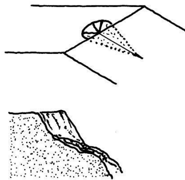
Fig. 38 Plateaurand an steilem Gehänge mit klufftbedingter Halbtrichter-Bildung
