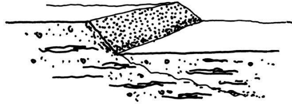
Fig. 85 Fluviale Terrasse: Wahrscheinlichere undeutliche Grenzlinie zwischen altem und neuem Schotterkörper
