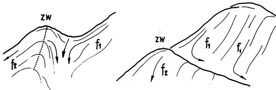
Fig. 101 Die Gehänge-Mulde, die das Gesamtgehänge trennt ZW Zwischenwasserscheide f 1 Falllinien, die von der Mulde abgelenkt werden f 2 Falllinien im unteren Gehängeteil
