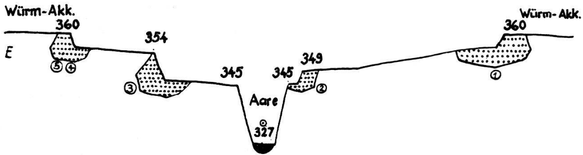
Fig. 87 «Querprofil Würenlingen–Villigen (halbschematisch). Aufschlüsse: 1 Kommetgraben Villigen (69), 2 Kommetgraben Villigen (68), 3 Zementfabrik Siggenthal (66), 4 und 5 Underfeld SW Würenlingen (64), (65). Die Geröllagen der tieferen Terrassenflächen ziehen unter dem höheren Terrassenhang durch und qualifizieren sie damit als Erosionsflächen.»
