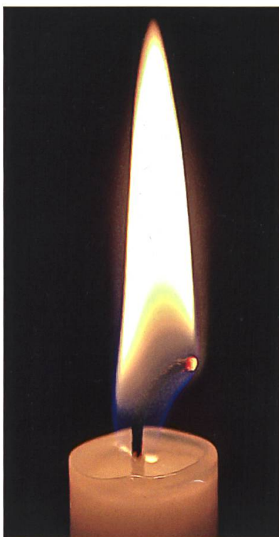
Abb. 4: Kerzenflamme: Im leuchtend hellen oberen Teil einer Kerzenflamme beträgt die Temperatur um die 1200^\circ\text{C} . Die am meisten Strahlungsenergie abgebenden Körper sind kleinste Russpartikel (schwarze Körper), die aus Millionen Kohlenstoffatomen bestehen, die mangels Sauerstoff noch nicht verbrannt sind. Die Entstehung dieser Russpartikel nahe beim Docht sieht man überzeugend nach dem Ausblasen der Kerze! Die maximale Strahlungsemission liegt für 1200^\circ\text{C} bei einer Wellenlänge von 2\mu\text{m} , also im infraroten Bereich. Deshalb erzeugt eine Kerze in erster Linie Wärme und nur relativ wenig sichtbares Licht. Bei den sichtbaren Wellenlängen emittiert sie am meisten Rot und fast kein Blau, deshalb ist das Kerzenlicht stark gelblich und «warm». Analog sind Flammen einer Petrollampe oder eines Feuers.
