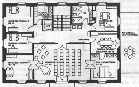
OBERGESCHOSS
