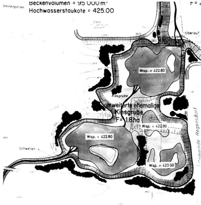
Im Vergleich das Vorlageprojekt 1987 (links) und das aufgrund der aktuellen Bestandesaufnahmen erarbeitete Gestaltungsprojekt 1992 (rechts) für das Areal der ehemaligen Kiesgrube «Gheid».
