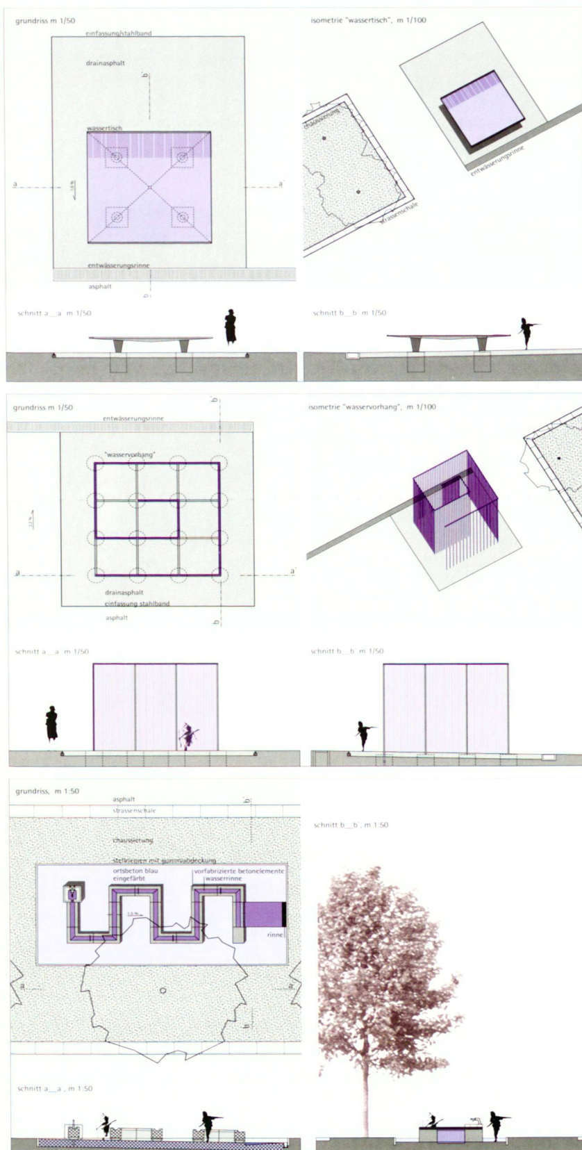
Talwiesen: Wassertisch (oben), Wasservorhang (Mitte), Wasserschlange (unten).
