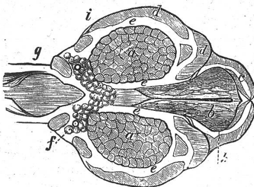
Fig. 21. — Section de thorax de mâle. — a , élévateur des ailes ; b , abaisseur des ailes ; c , antagoniste de l'abaisseur ; d , muscles de l'aile postérieure ; e , sacs à air ; f , système de glandes n° 3 ; g , cou ; h , mésophragme ; i , stigmates.
