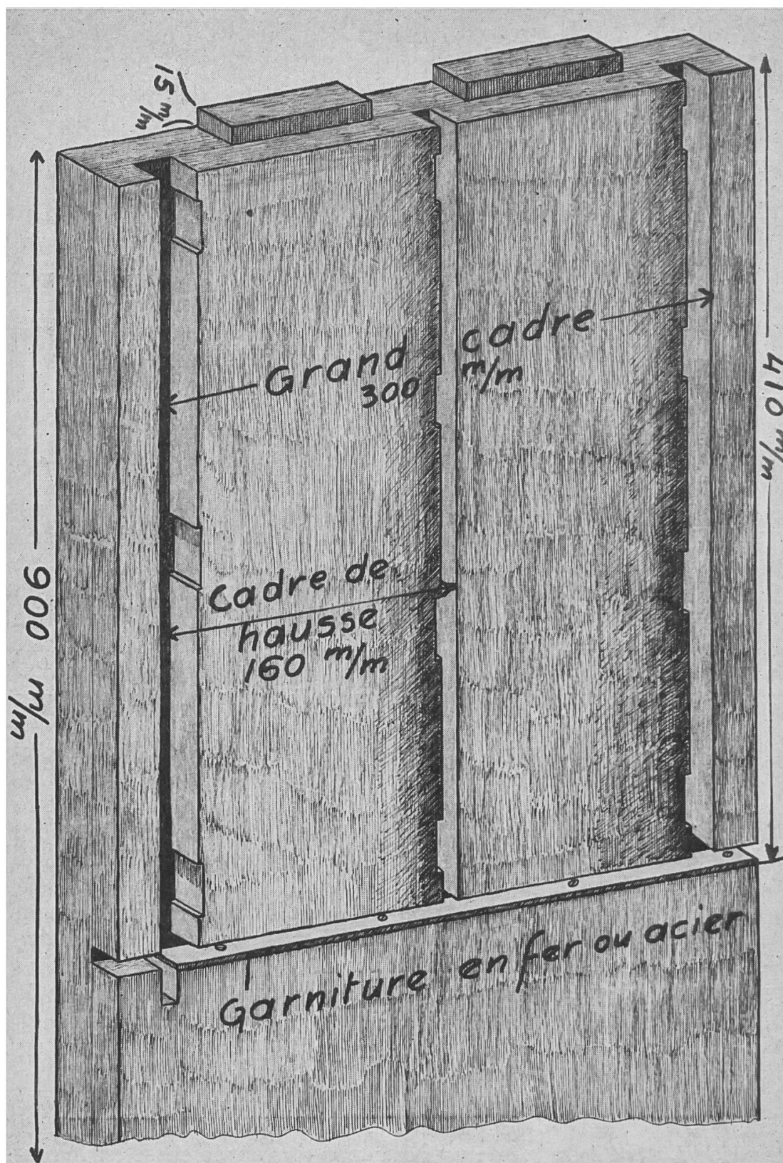
GABARIT POUR CADRES « DADANT-BLATT »
