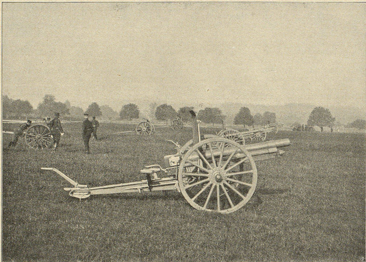
Geschütz in Ruhstellung.
