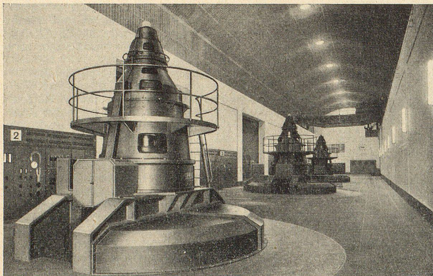
Innenansicht der Zentrale mit den drei vorläufig eingebauten Maschinengruppen und ihren Bedienungs- und Kontrollinstrumenten.
