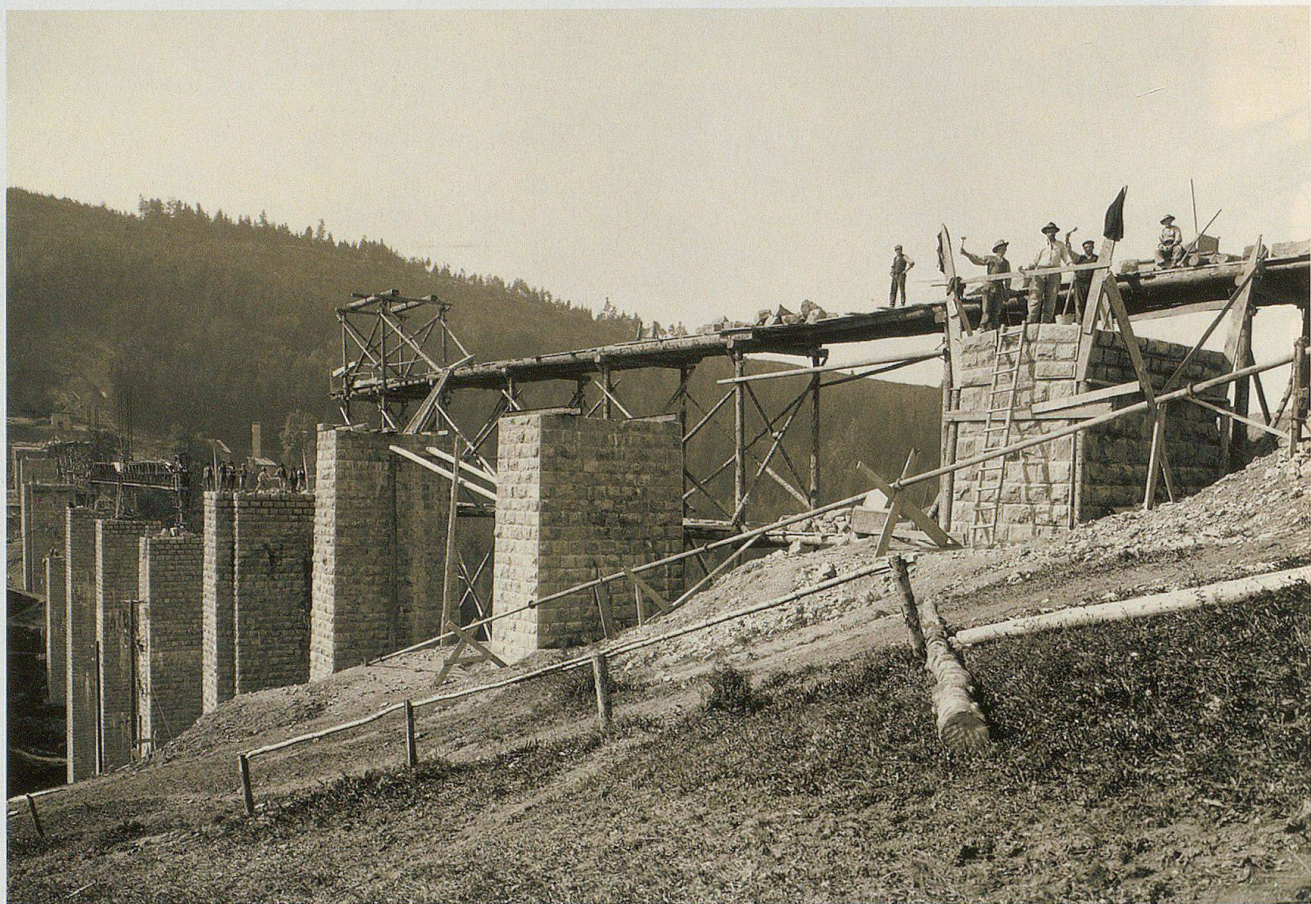
Der 289 Meter lange und 64 Meter hohe Wissenbach-Viadukt zwischen Herisau-Schachen und Degersheim.
