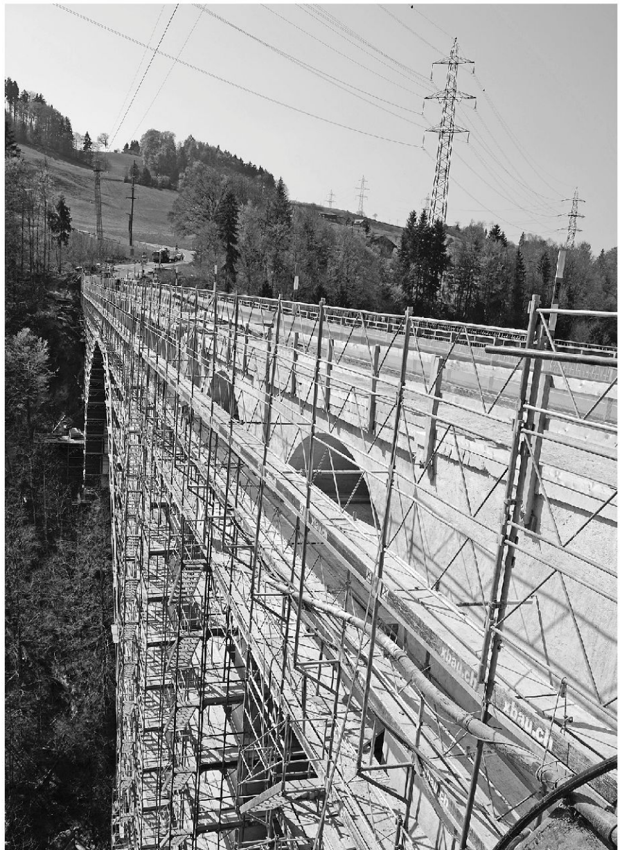
Sanierung im Jahre 2011.
