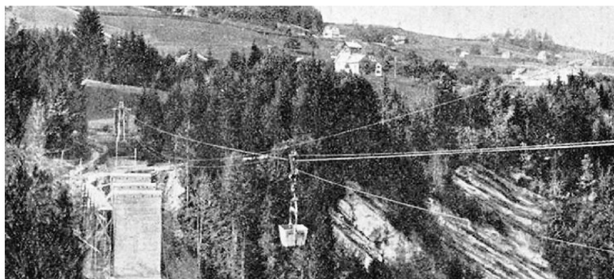
Betonbeförderung mit der Schwebeseilbahn.
