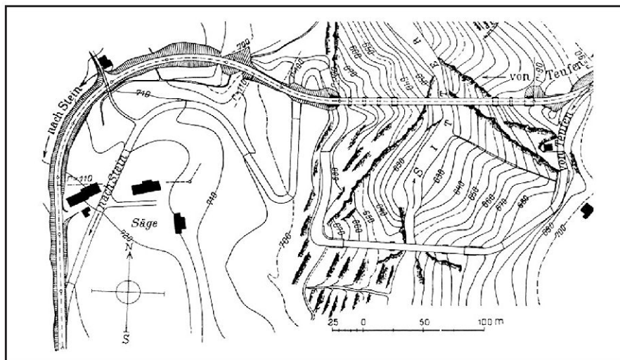
Lageplan mit alter und neuer Brücke.
