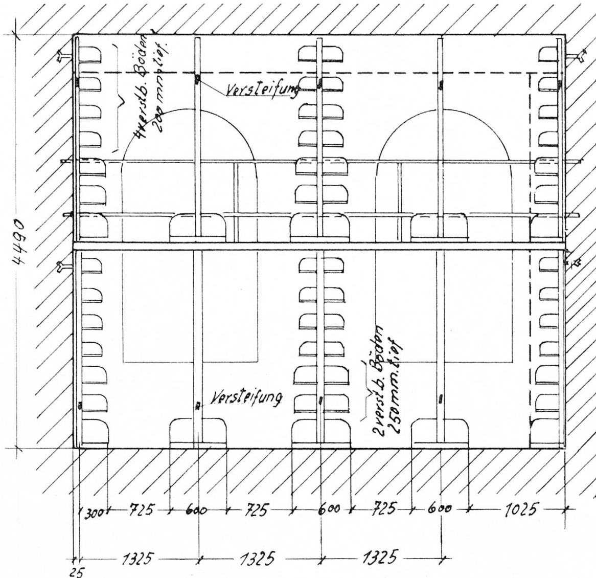
Schnittzeichnung einer 2-geschossigen Bibliothekanlage in einem Altbau
