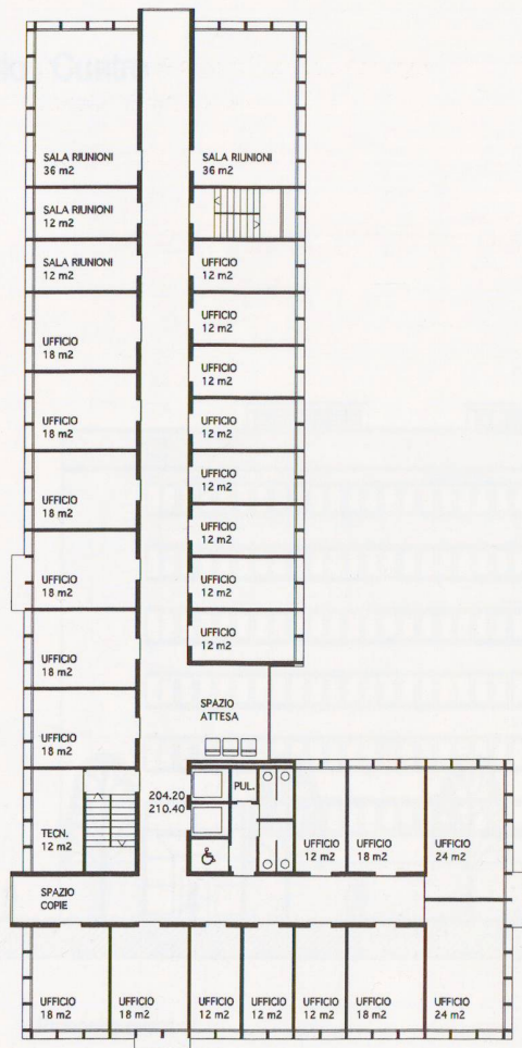
Pianta piano tipo
